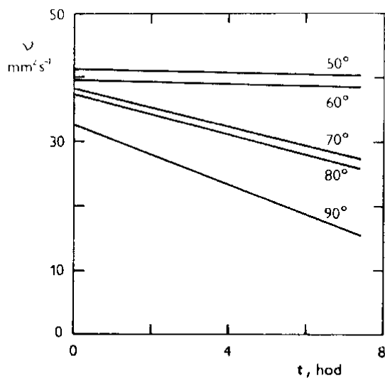
Obr. 13 Závislost kinematické viskozity \eta na době zahřívání t při různých teplotách vodného roztoku kožního klišu ^{\circ} .
