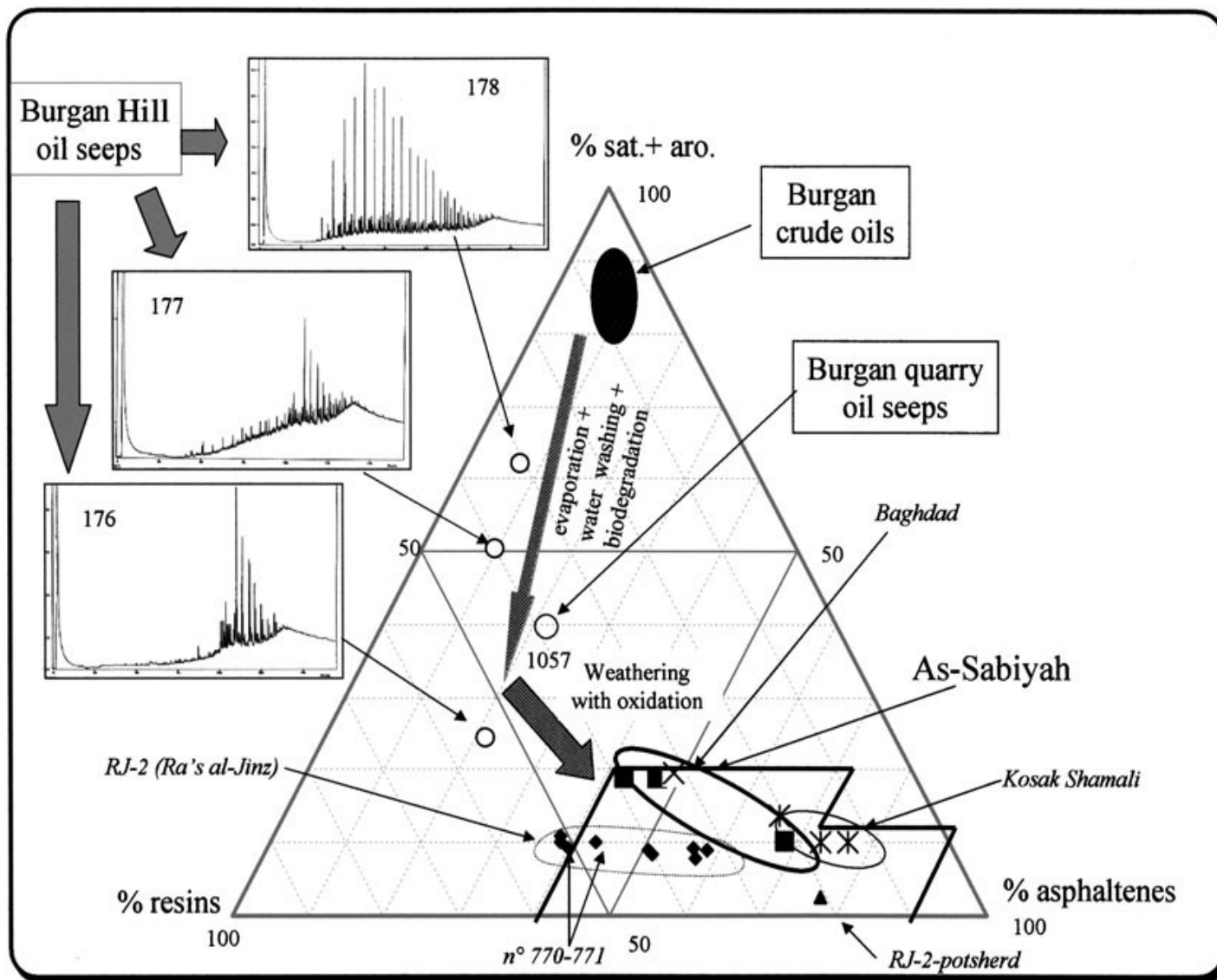
Ternární diagram hrubého složení organických látek extrahovaných chloroformem nebo dichlormethanem ("nasycené + aromatické látky", "pryskyřice" a "asfalteny"), který poskytuje srovnání mezi vzorky bitumenu z As-Sabiyah, Ra's al-Jinz, Bagdádu a Kosak Shamali a ropnými průsaky a surovou ropou z Burganu (Kuvajt).
