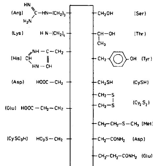
Obr. 2-28. Reaktívne miesta bočných reťazcov aminokyselín v keratine vlny
