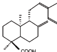
ozic acid
