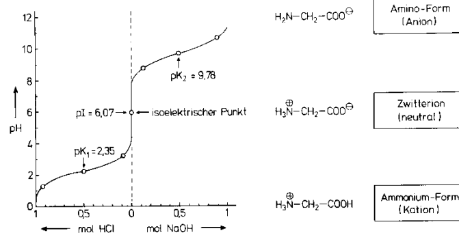
Abb. 11.2 Titrationskurve der α-Aminosäure Glycin. (Als Zeichenhilfe wurden auch die pK ± 1-Werte bei 0,1 und 0,9 mol Lauge oder Säure eingezeichnet)
