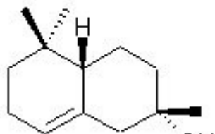
alpha-ambrinol
