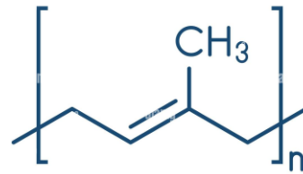
trans -polyisoprene
