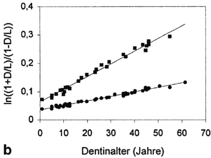
Abb. 1a,b ◀ Razemisierungsgrad von Asparaginsäure (als \ln[(1+D/L)/(1-D/L)] ; D/L=D - L -Asparaginsäure) in Gesamtdentin (Kreise) und der säurelöslichen Dentinproteinfraktion (Quadrate) in Abhängigkeit vom Dentalter: a im deutschen Kollektiv, b im türkischen Kollektiv
