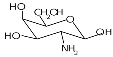
galaktosamin- ^4C_1
