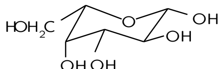
\beta -L-galaktopyranosa- ^1C_4
