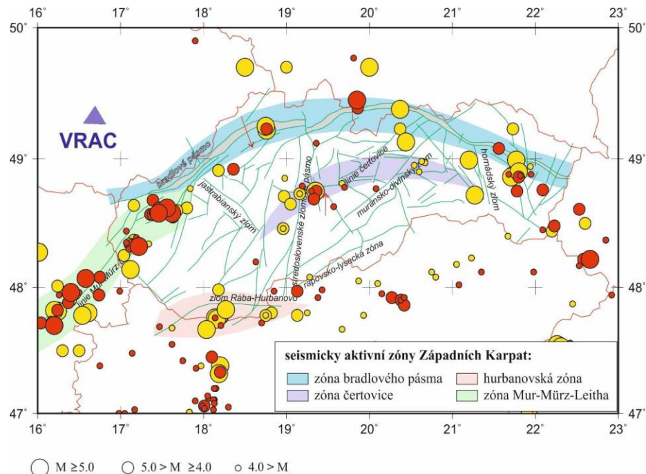
Epicentra historických otřesů z let 1590-1899 (žlutá kolečka) a 1900-2006 (červená kolečka).
