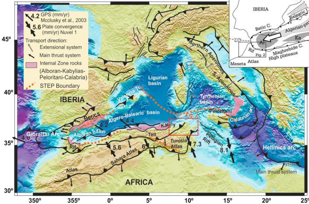
Tektonické schéma západní části Středomořího moře (Booth-Rea et al. 2018)
