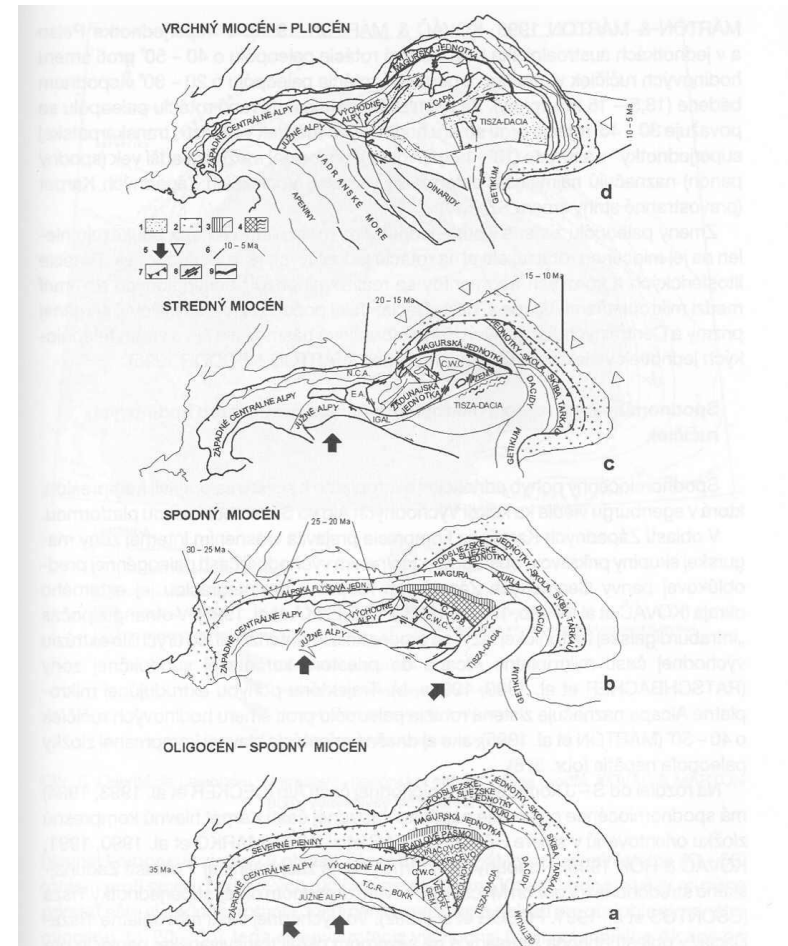
Obr. 4. Palinspastická rekonštrukcia neoalpínskeho vývoja alpsko-karpatsko-panónskej oblasti. Zostavené na základe prác BALLA (1984, 1987), JIŘÍČEK (1979), HORVÁTH (1984), KOVÁČ et al. (1989a, 1994a), ROYDEN (1988), SANDULESCU (1988), SEIFERT (1992). Vysvetlivky: 1 – neogénne panvy, 2 – čelná predhľeba, 3 – bradlové pásmo, 4 – szolnocký flyšový bazén, 5 – orientácia hlavnej kompresie, 6 – posledné dosnutie príkrovov na platformné predpolie, 7 – násuny príkrovov, 8 – horizontálne posuny; ďalšie vysvetlivky na strane 13.
