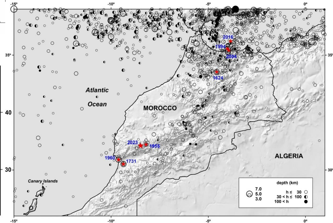
Seismicita Maroka (Peláez 2023, Temblor)
