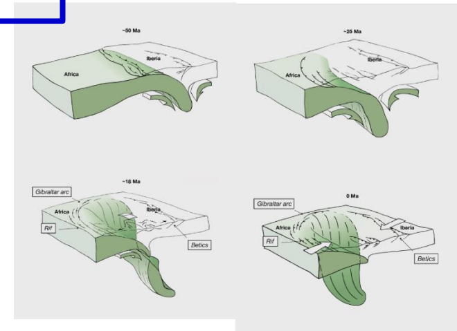
Vývoj Gibraltarského oblouku podle Joliveta
