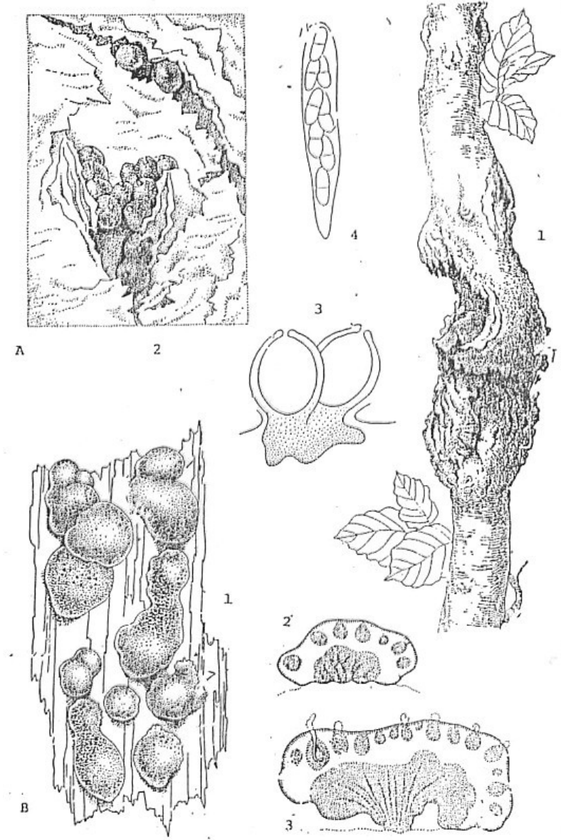
Obr. 58: Hypocreales .
