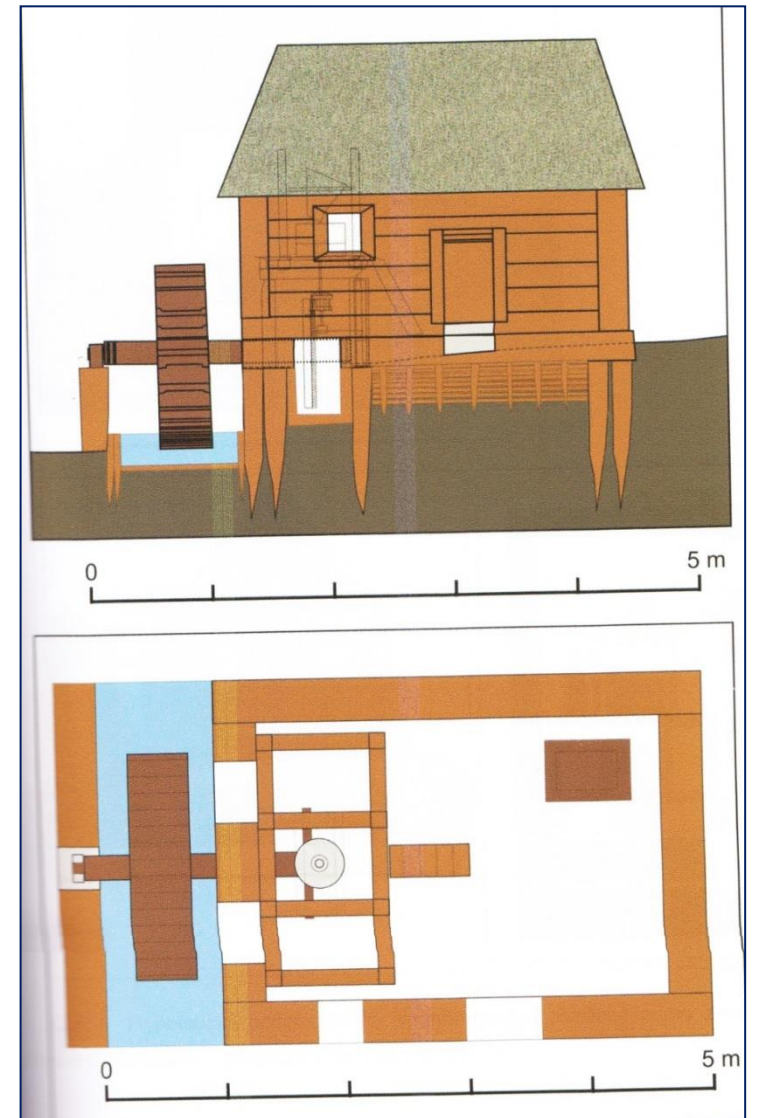
Rekonstrukce vodního mlýna podle Lucie Galusové
