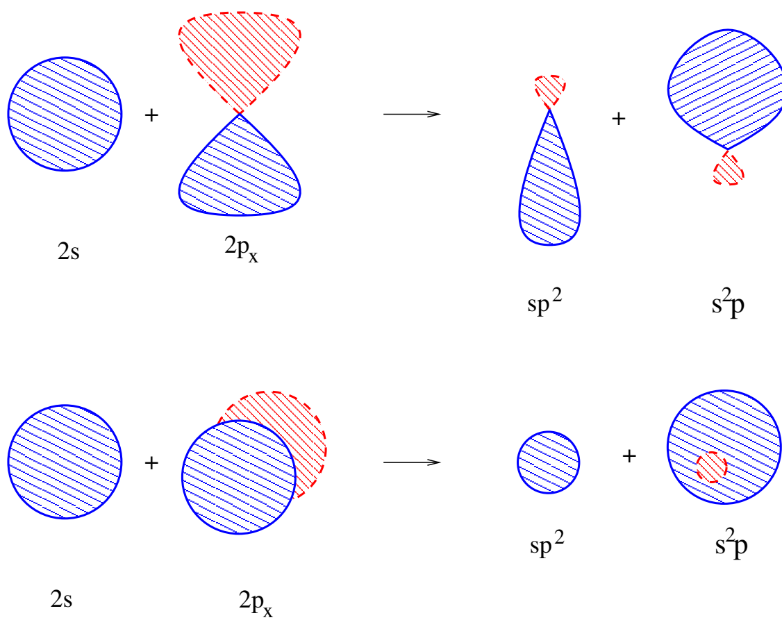
Obrázek 19.3: Orbitaly sp^2
