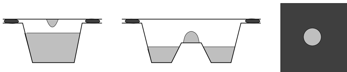
Obrázek 12.6: Krystalizační metody visící kapky (vlevo), sedící kapky (uprostřed) a mikrodávek (vpravo).
