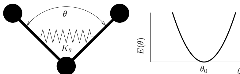
Obrázek 11.2: Zjednodušený popis energie spojené s deformací vazebného úhlu.
