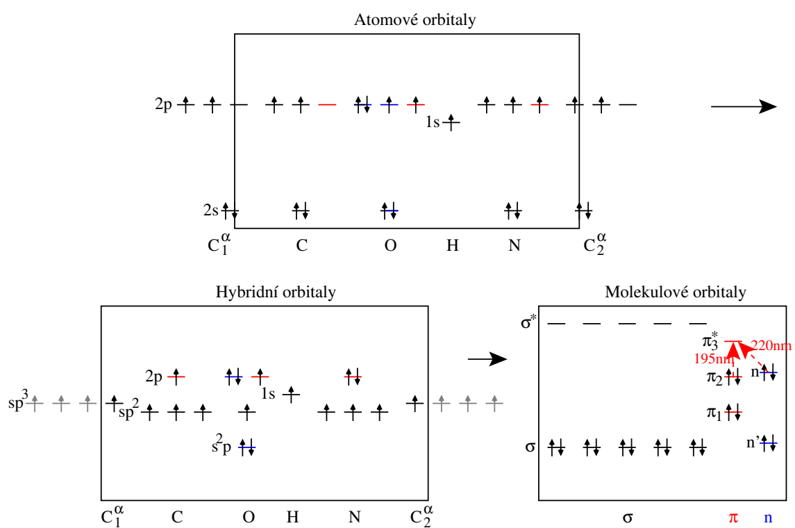
Obrázek 19.6: Energetické rozložení orbitalů peptidové skupiny.
