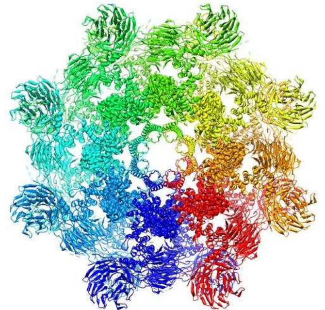
apoptosom
