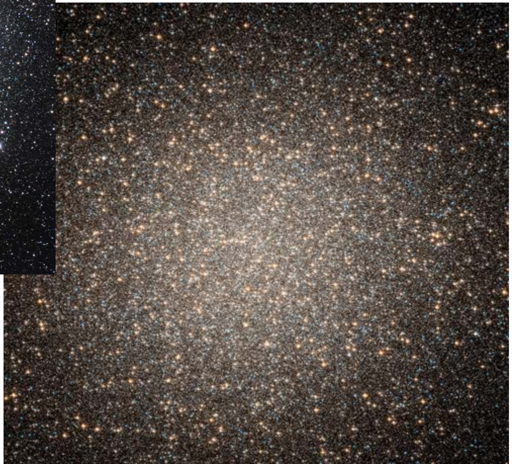
10' střed Omega Centauri (HST)
