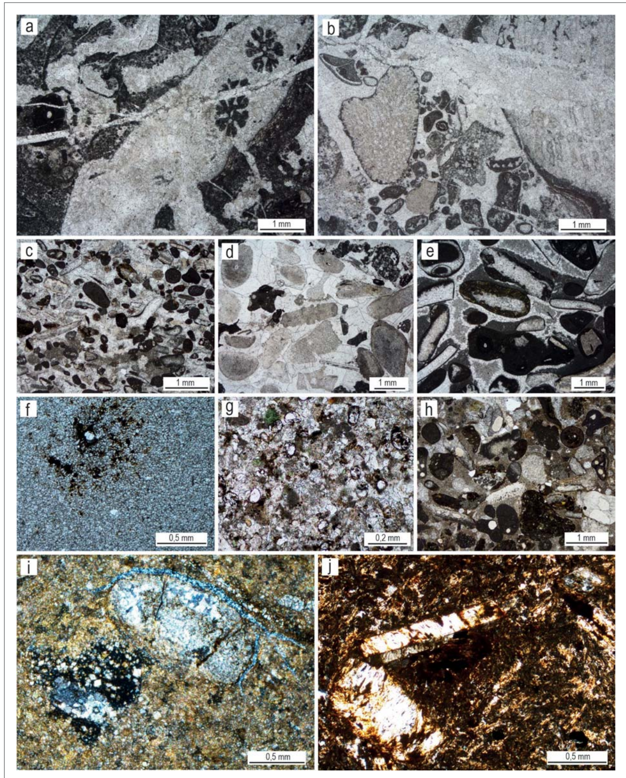
Obr. 5: Klasty ze slepenců, Starý Jičín – hradní příkop: a – částečně rekrystalovaný pelmikit s korálem a mikrobiálními povlaky v růstové pozici (bafflestone?), MB135-E; b – čočka biodetritického floatstone v biopelmikritu (vlevo dole), MB135-F; c – částečně rekrystalovaný biointramikrit (wackestone), MB135-C; d – krinoidový biosparit; MB135-B; e – intrabiomikrit s kortoidy (wackestone), MB135-D; f – dolomitizovaný biomikrit, MB135-I; g – jemnozrný písčítý vápenec s jehlicemi hub a glaukonitem, MB135-H; h – hrubozrný detritický vápenec s bodovou silicifikací (světlé tečky), MB135-G; i – dolomitický vápenec s jílovitými enklávami a rekrystalovaným bioklastem? ohraničeným cirkumgranulární trhlinou, MB135-A; j – alterovaný trachyt s vyrostlící plagioklasu, MB135-K.
