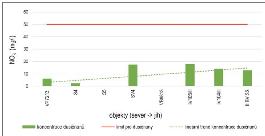
Obr. 3: Obsah dusičnanů v podzemní vodě kolektoru B. Fig. 3: Nitrate content in groundwater of aquifer B.
