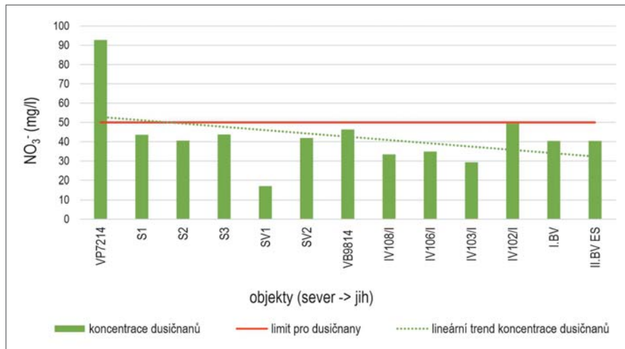
Obr. 2: Obsah dusičnanů v podzemní vodě kolektoru C. Fig. 2: Nitrate content in groundwater of aquifer C.
