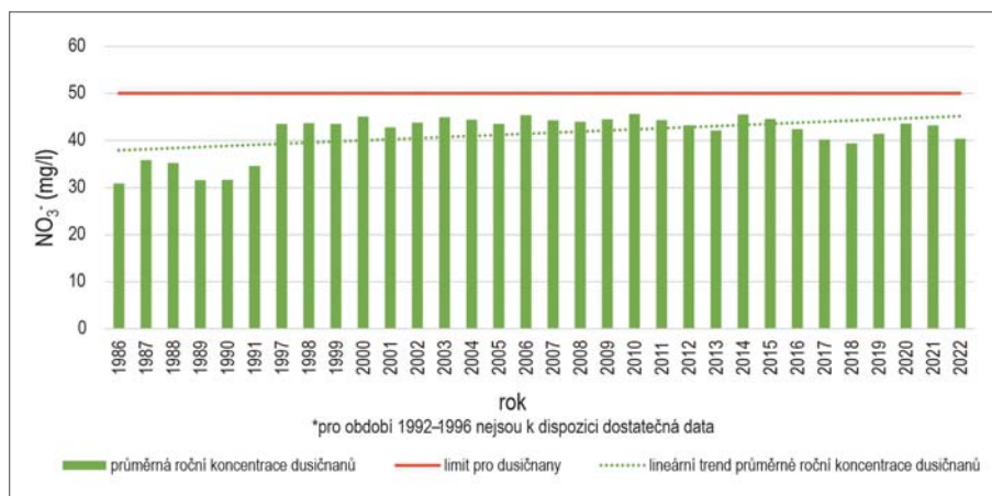
Obr. 4: Obsah dusičnanů v podzemní vodě I. březovského vodovodu. Fig. 4: Nitrate content in groundwater of I. Březová water main.
