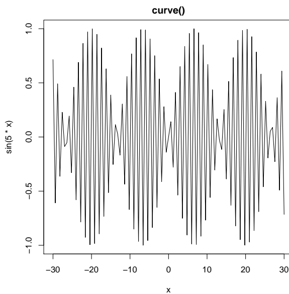
Obr. 7.14. Funkce curve()
