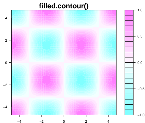
Obr. 7.18. Funkce filled.contour()
