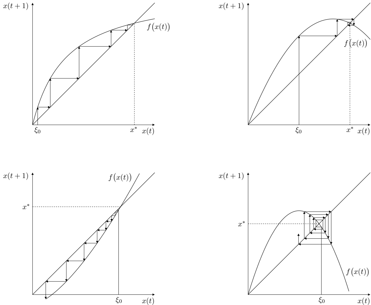
Obrázek 4.2: Grafické řešení autonomní rovnice (4.7). Vlevo „schodový diagram“, vpravo „pavučinový diagram“, nahoře stabilní (přitahující) pevný (rovnovážný) bod zobrazení f , dole nestabilní (odpuzející).
