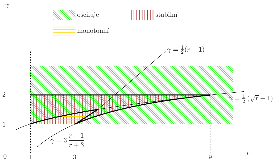
Obrázek 6.6: Závislost kvalitativních vlastností řešení systému (6.94) (modelu dravec-kořist J. Maynarda Smithe) v okolí vnitřního stacionárního bodu (koexistenční rovnováhy) na hodnotách růstového koeficientu kořisti r a „efektivity predace“ \gamma .
