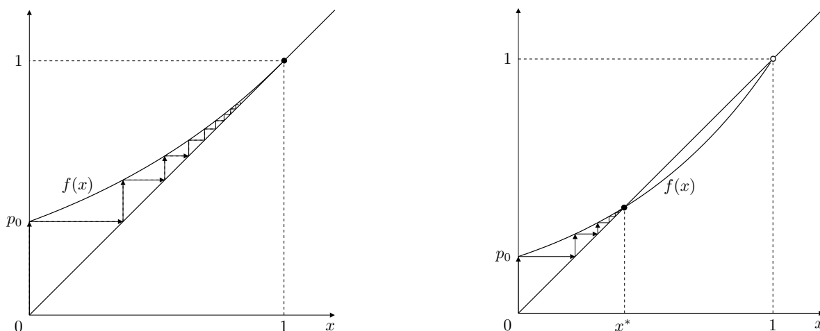
Obrázek 6.4: Graficé řešení počáteční úlohy (6.61), (6.56) v případě f'(1) \leq 1 (vlevo) a f'(1) > 1 (vpravo).
